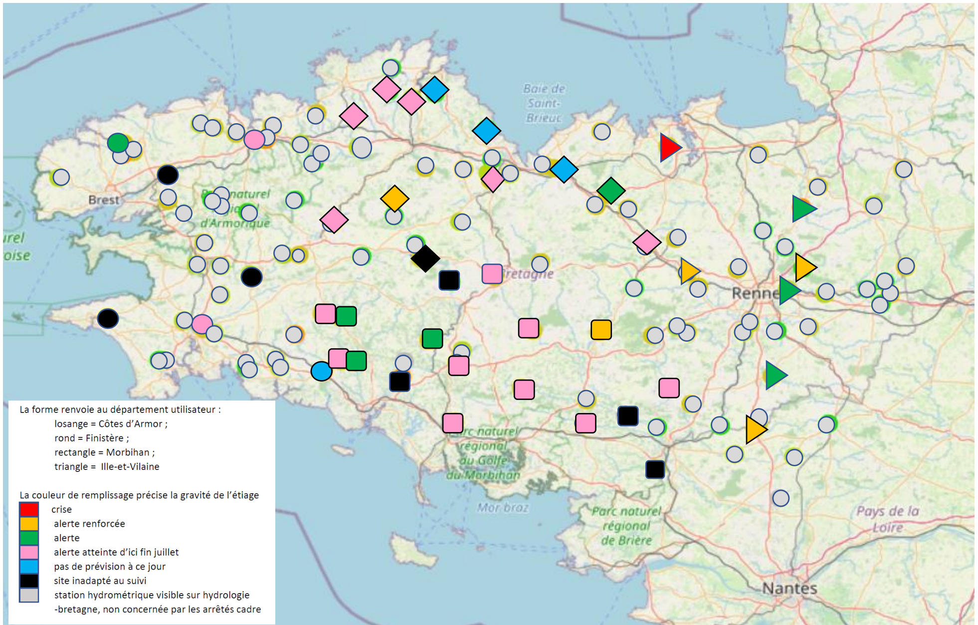
Etat au 14 juillet 2022 des rivières servant de repère pour les arrêtés préfectoraux de gestion des étiages
